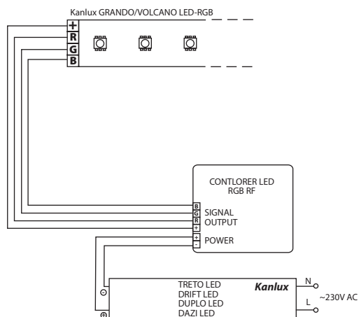
LED RGB line modules feed system and colour controlling wiring diagram Ein Beispielschema für die Energieversorgung und Farbensteuerung der LED RGB Linienmodule
